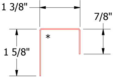
MPA270-J Closure
