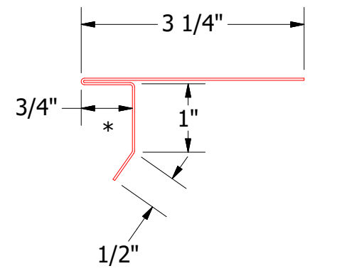
HSA112-Drip Edge
