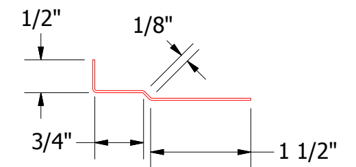
Joggle Cleat
